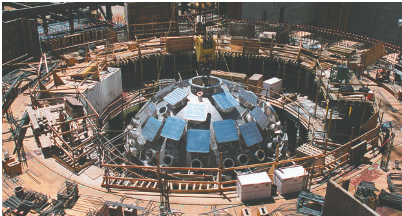
Строительство Международного термоядерного реактора
